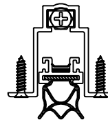
PEMKO 434APKL AUTOMATIC DOOR BOTTOM
